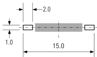
Löt pads
