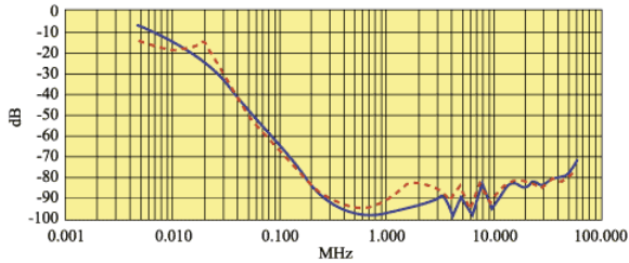
FL 155.10.00 10 A
