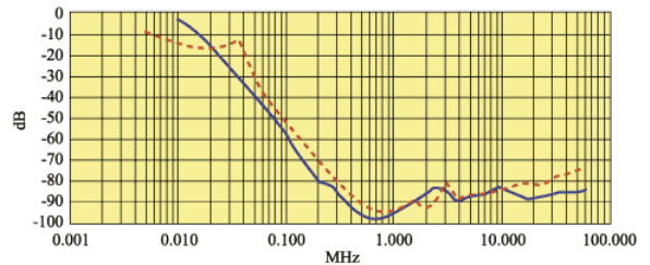
FL 155.30.00 30 A
