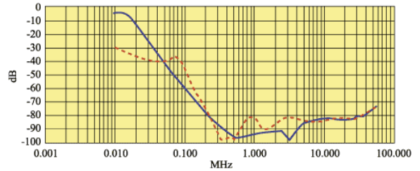
FL 155.120.00 120 A
