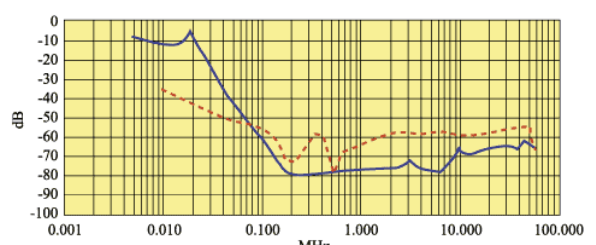
FL 155.300.00 300 A
