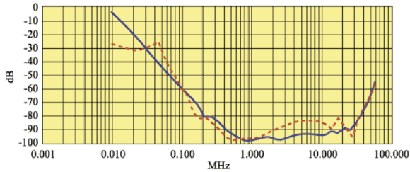
FL 155.80.00 80 A
