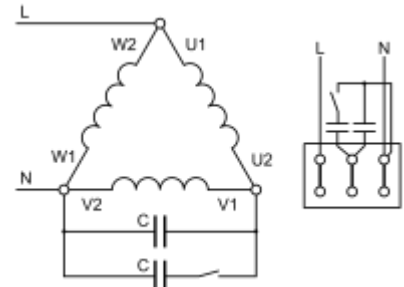
Steinmetz-Schaltung im Dreieck mit Anlauf-Kondensator
