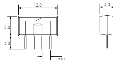
MK mit integriertem Widerstand
