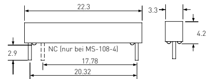
MK mit integriertem Widerstand
